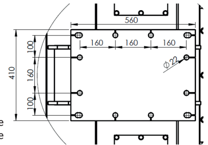
Anschlußmaße Kopfplatte für Terra-Star® Compactline
