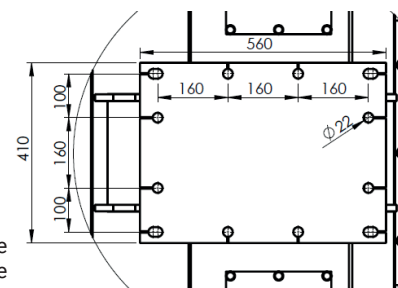
Anschlußmaße Kopfplatte für Terra-Star® Compactline
