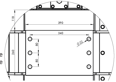
Anschlußmaße Kopfplatte für Terra-Star® Ecoline
